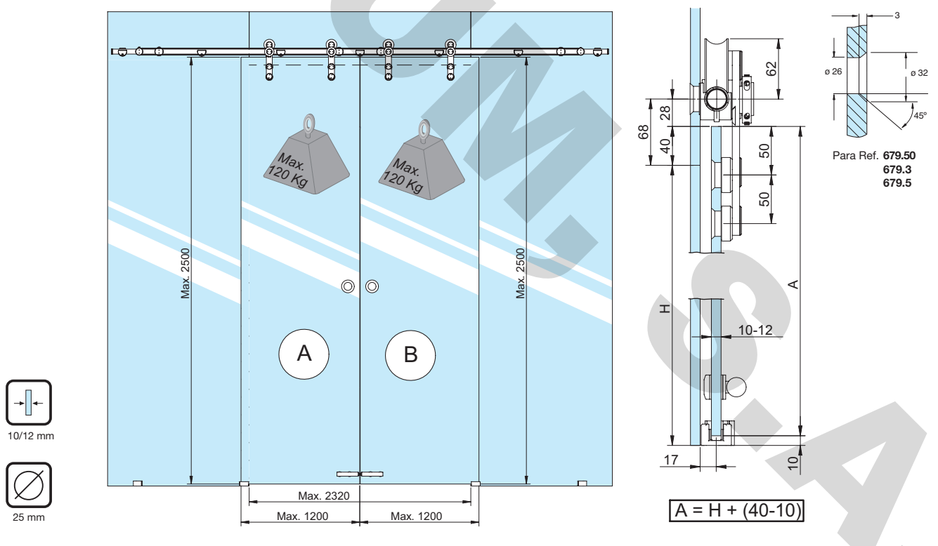
Alzado y sección tipo (Cotas en mm)
