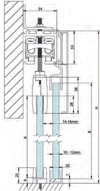
MONTAJE A PARED VIDRIO FIJO
