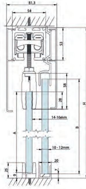
MONTAJE A TECHO VIDRIO FIJO
